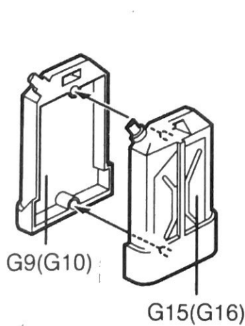
ISRAELI JERRY CAN 이스라엘 제리캔
