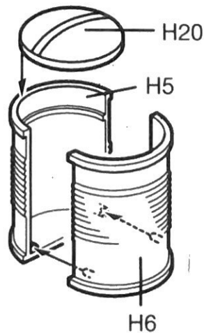
U.S. HOT/COLD DRINK CONTAINER 미군 보온 식수통
