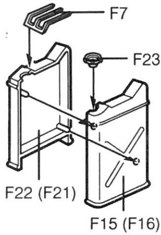
U.S. JERRY CAN 미군 제리캔
