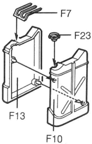
U.S. JERRY CAN 미군 제리캔
