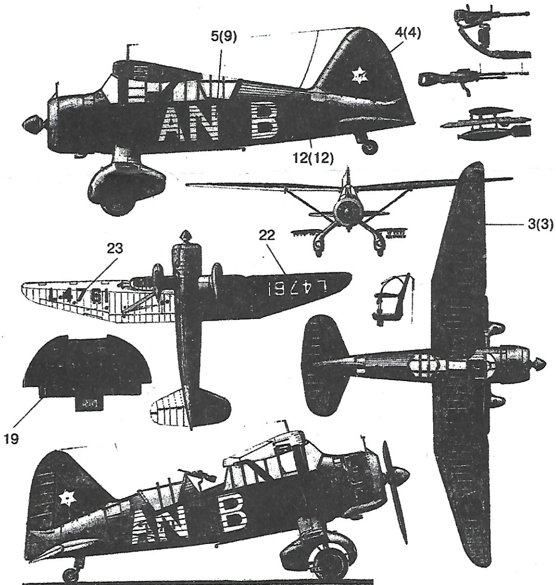
Лизандер Mk III КВС Великобритании. 1940 г. Westland Lysander Mk III of R.A.F. 1940
