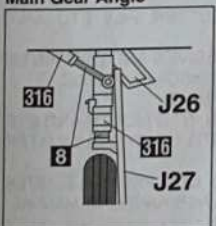
主脚の組み立て 参考図 Main Gear Angle
