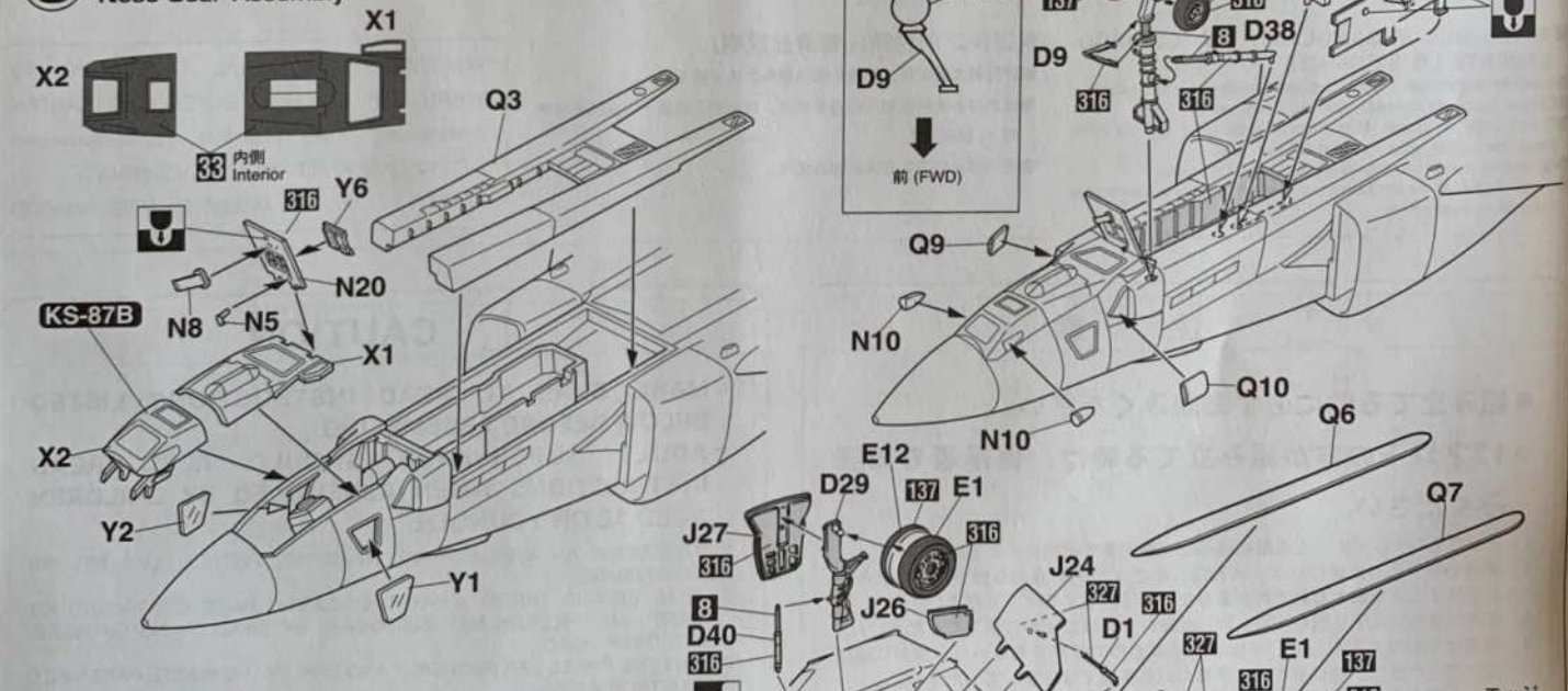
主脚の組み立て 参考図 Main Gear Angle
