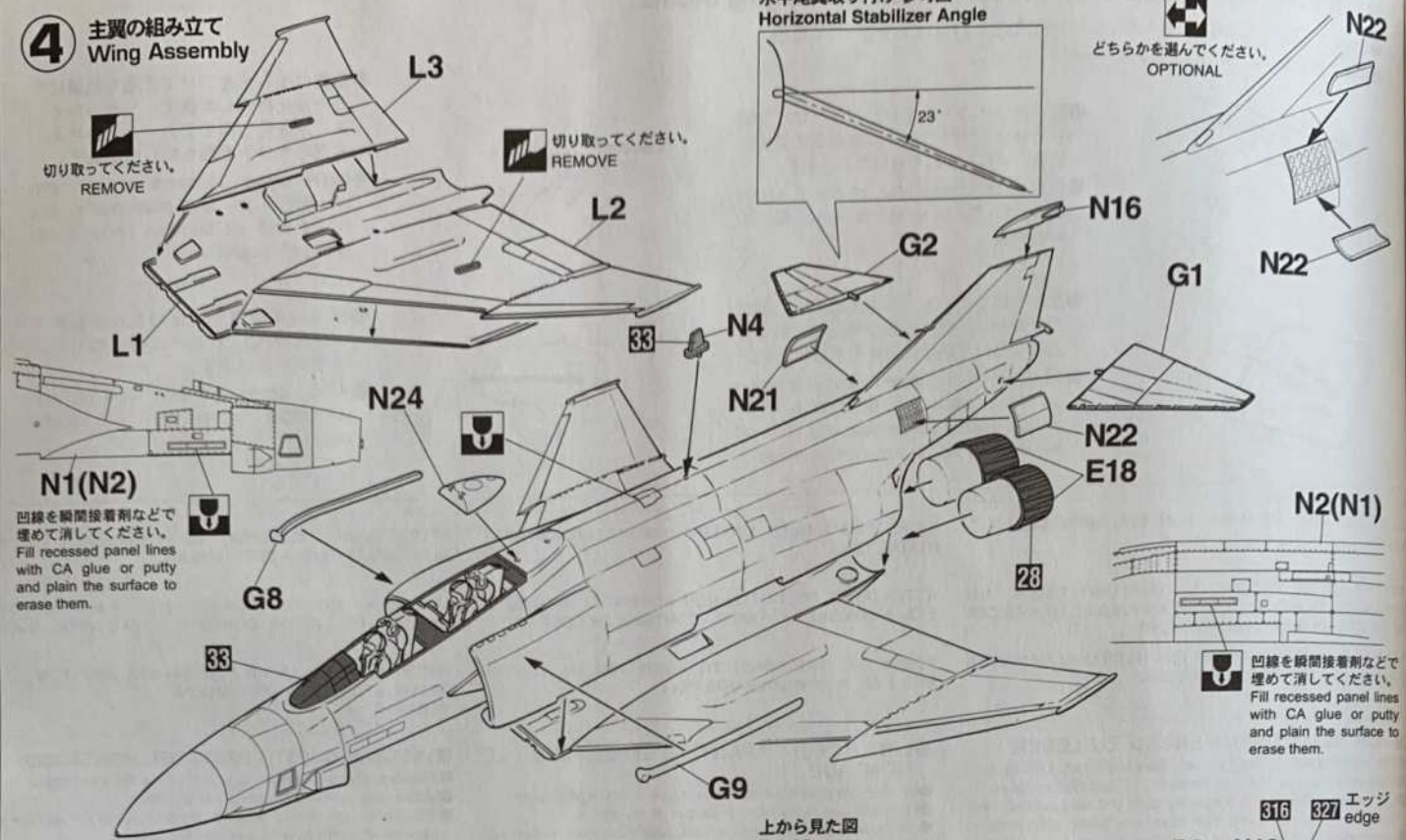
上から見た図 Top View
