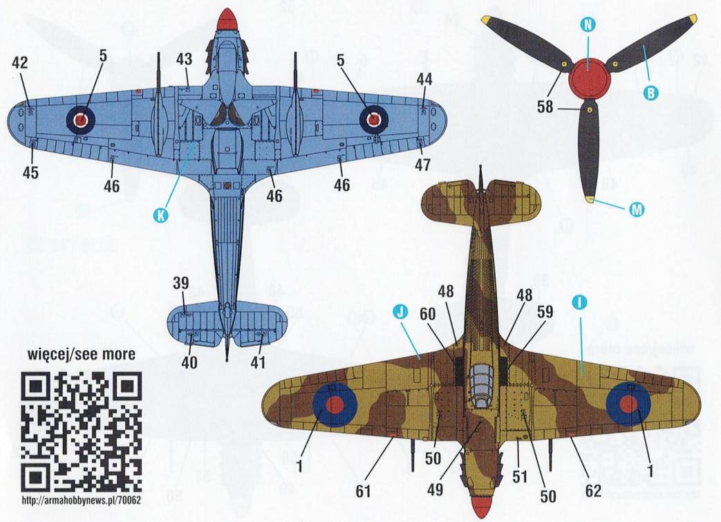
Hurricane Mk.IID Trop, KW704/R „Christine”, 6. Dywizjon RAF, lotnisko Gabes, Tunezja, kwiecień 1943 r. Pilot F/O A.H.M. Clarke. Hurricane Mk.IID Trop, KW704/R „Christine”, No. 6 Squadron RAF, Gabes, Tunisia, April 1943. Pilot F/O A.H.M. Clarke.
