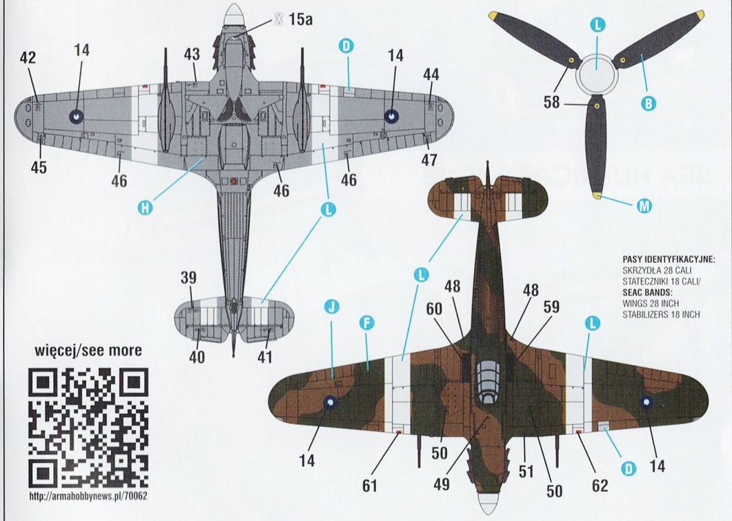
Hurricane Mk.IID Trop, HW874/X, 20 Dywizjon RAF, lotnisko Monywa, Birma, wiosna 1945 r. Hurricane Mk.IID Trop, HW874/X, No. 20 Squadron RAF, Monywa, Burma, spring 1945.
