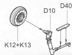
《左侧主起落架》 Left main undercarriage
