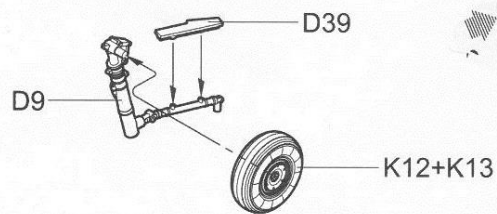
《右侧主起落架》 Right main undercarriage
