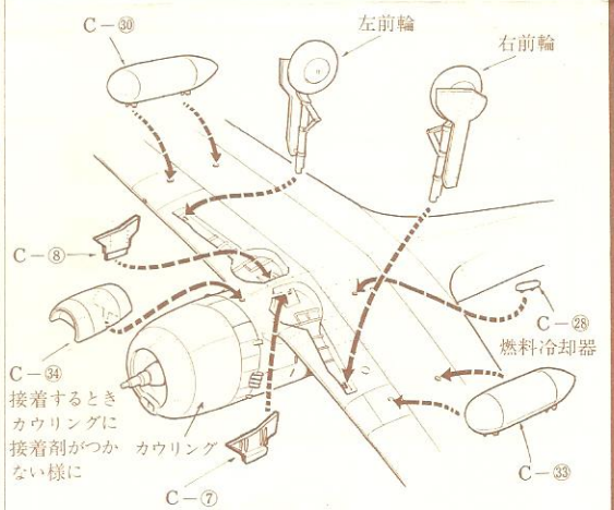
11 各部品を接着しましょう。
