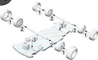
车轮及底部拼装图
