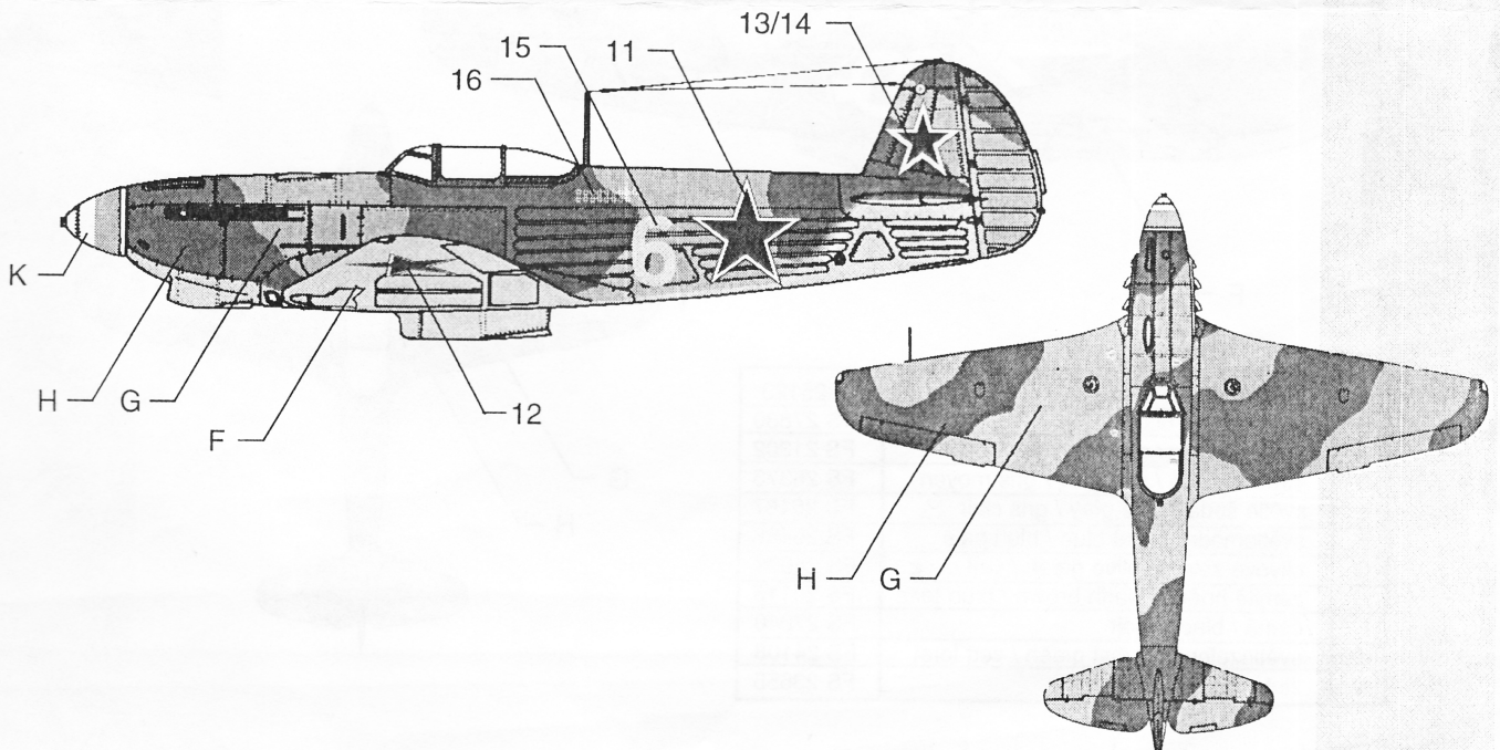
Jakovlev Jak-9 por. Marcel Albert (23 vítězství, Hrdina Sovětského svazu), Antonovo, říjen 1944 Lt. Marcel Albert (23 kills, Hero of Soviet Union), Antonovo, October 1944 Lt. Marcel Albert (23 victoires) Antonovo, Octobre 1944
